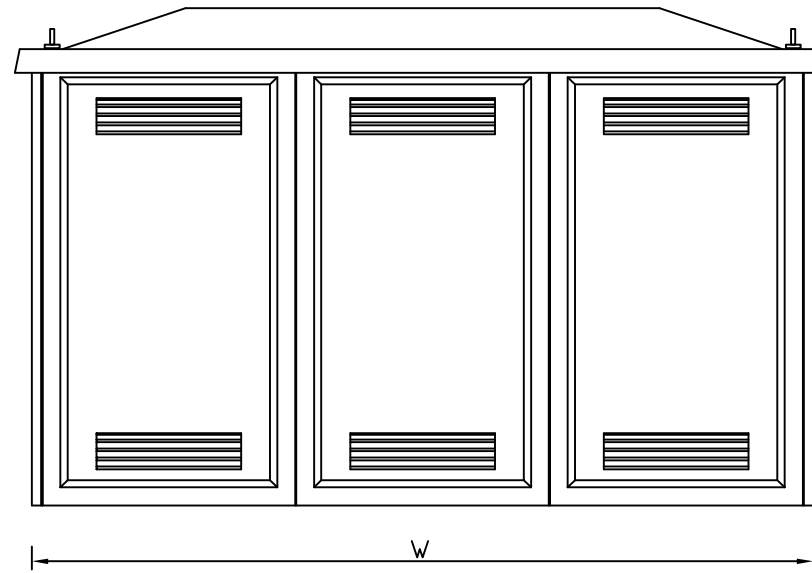
TYP. SIDE ELEVATION
